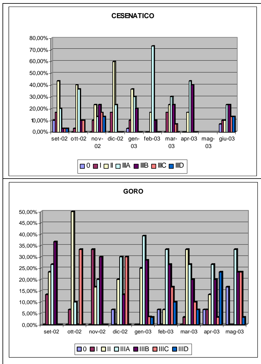
Grafico 56 - Percentuali delle classi Lubet nelle tre stazioni di campionamento
