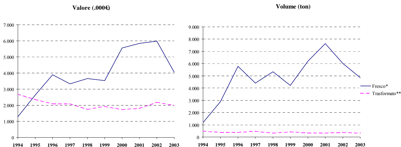
Grafico 13 - Evoluzione e composizione delle esportazioni italiane di mitili
