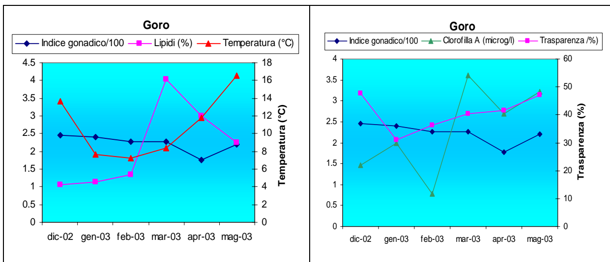
Grafico 59 - IG (riportato come IG/100) rispetto a Temp., Lipidi, Clorofilla A e Trasparenza in località Goro
