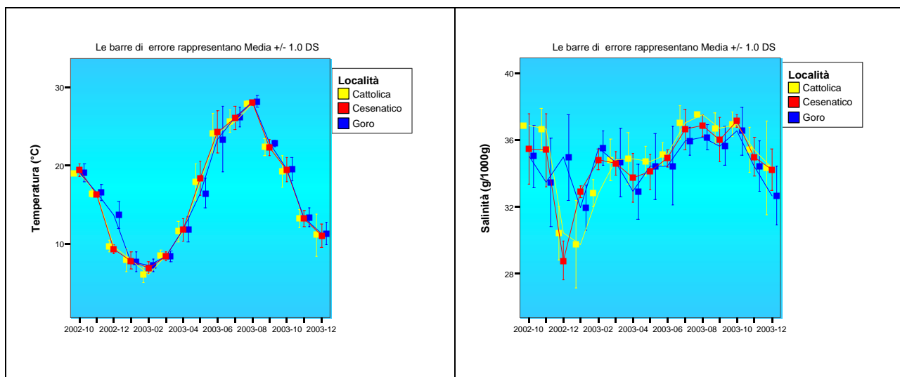
Grafico 60 - Andamento medio mensile della temperatura e della salinità nelle tre località
