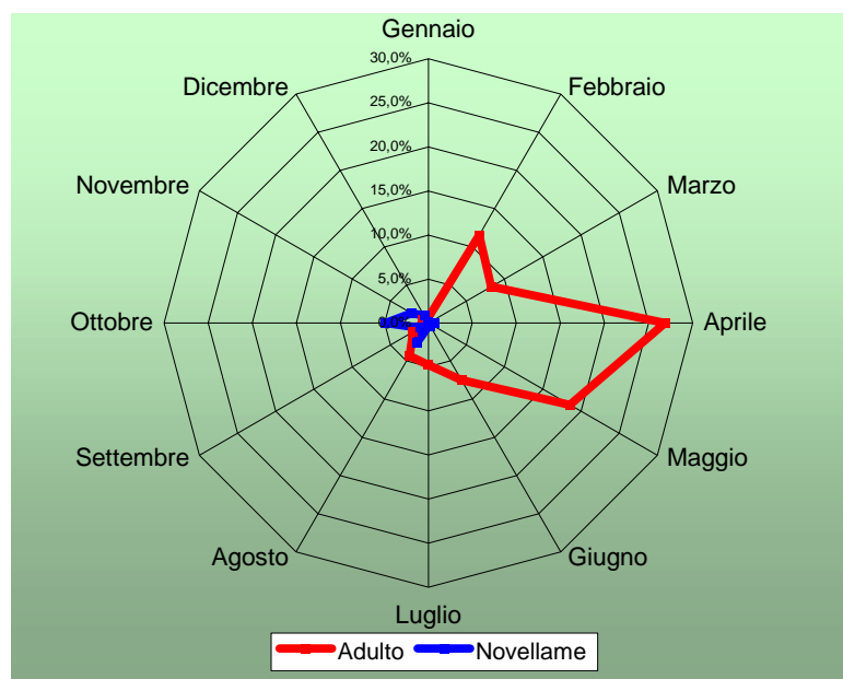
Grafico 36 - Andamento della commercializzazione mensile di mitili per l'anno 2002 nelle componenti adulto e novellame
